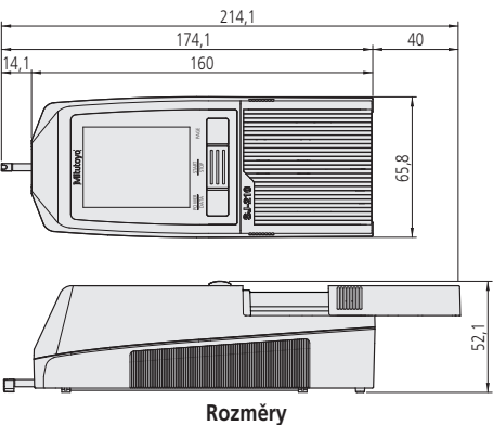
Rozměry
